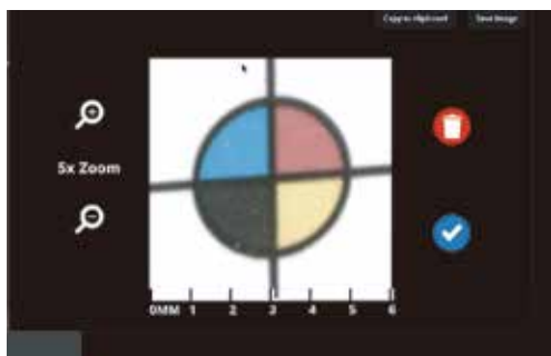
图3： 在该套准线上使用5倍变焦显示，黄色溢出到套准圆以外；没有数字放大镜功能将无法发现这个问题。
